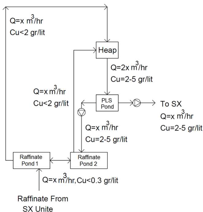
شکل ۲- فلودیگرام طراحی گردش جریان های PLS و رافینت در بین واحدهای هیپ و SX پروژه لیچینگ سونگون
