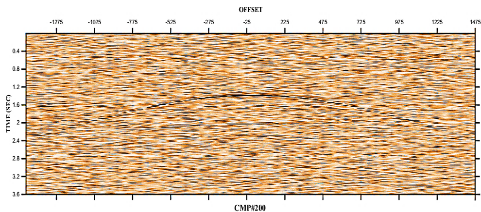
شکل ۵- مقطع نقطه میانی مشترک شماره ۲۰۰.
