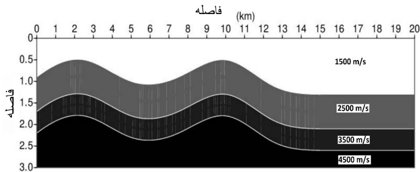
شکل ۱- مدل سرعت مصنوعی ایجاد شده در نرم افزار ساینمیک یونیکس
