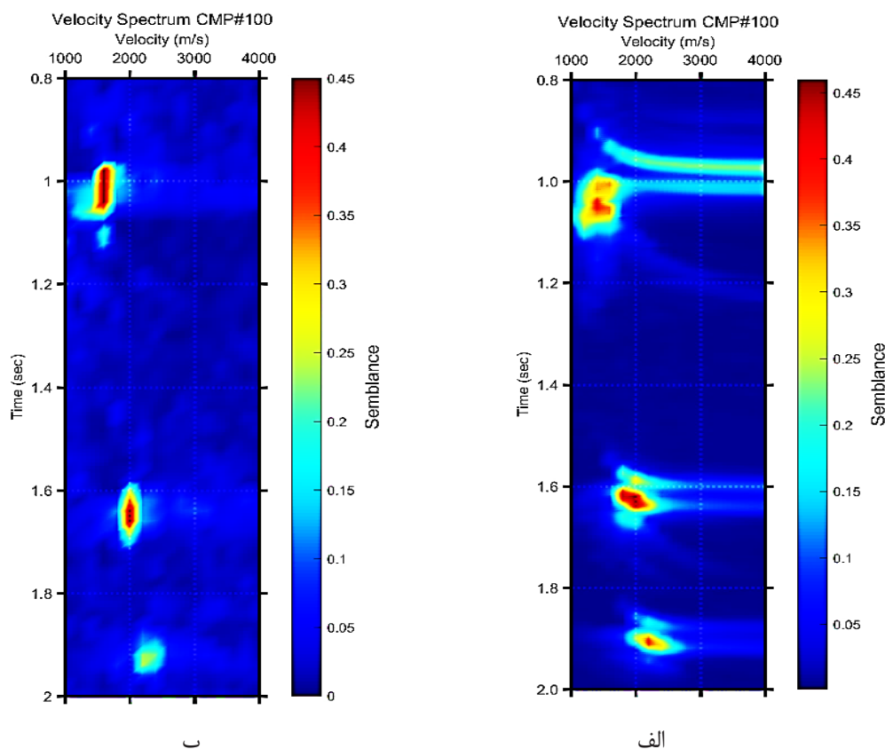
شکل ۳- الف) مقطع طیف سرعت حاصل از روش پیشنهادی، ب) مقطع طیف سرعت حاصل از روش معمول
