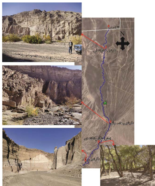
شکل ۵- انواع ناپیوستگی‌ها و دگرشیبی‌ها در طول دره راگه و جایگاه آنها در عکس هوایی و بانمای صحرایی از آنها. همچنین موقعیت بهترین استراحتگاه یا تفرجگاه پادگان‌های بر روی شکل نشان داده شده است.
